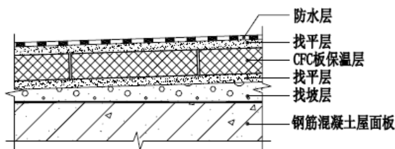
图 C.0.2 CFC 板屋面保温基本构造
