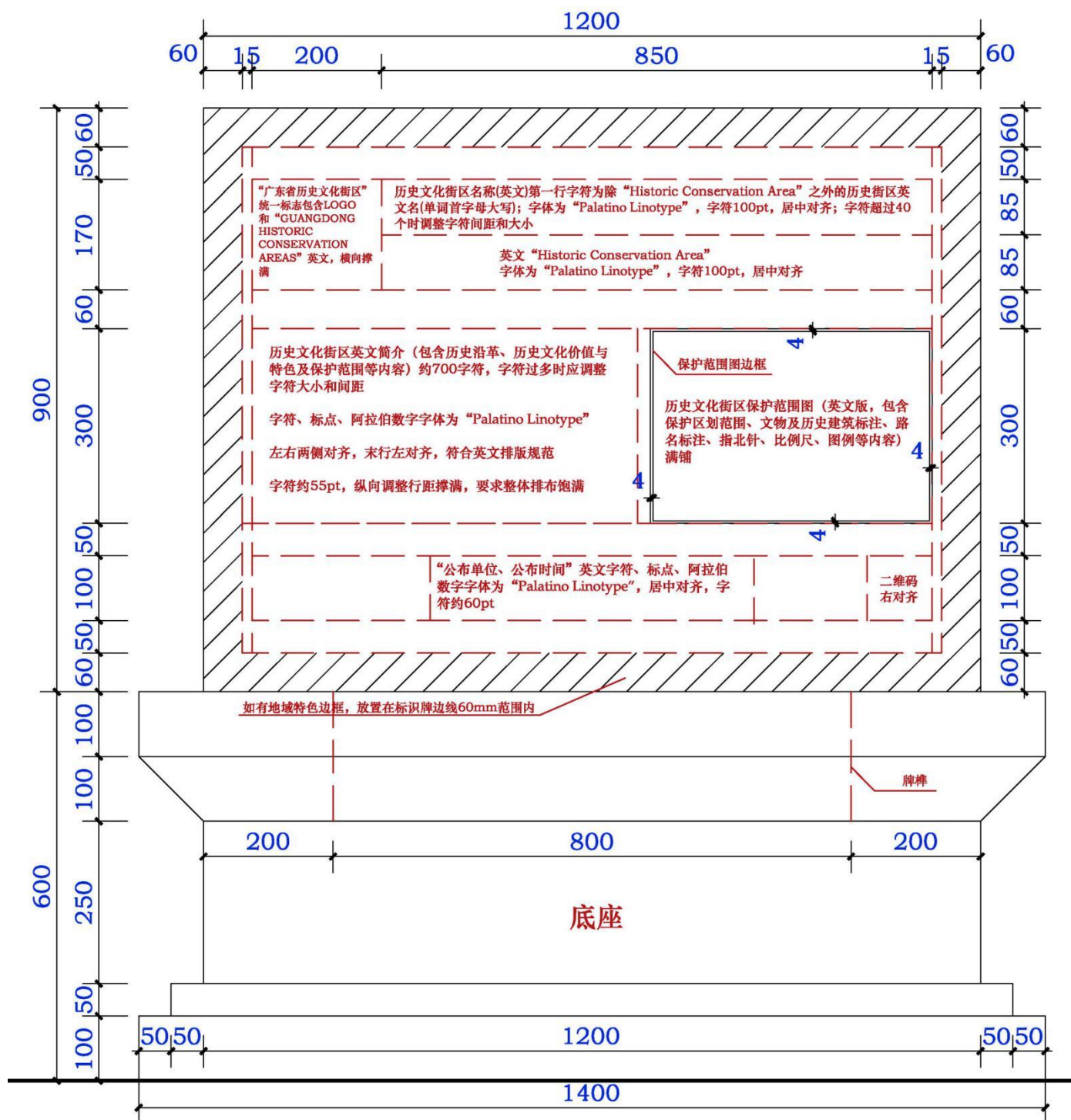
图 2: 保护标志牌排版规则、安装高度示意图 (横版背面)
