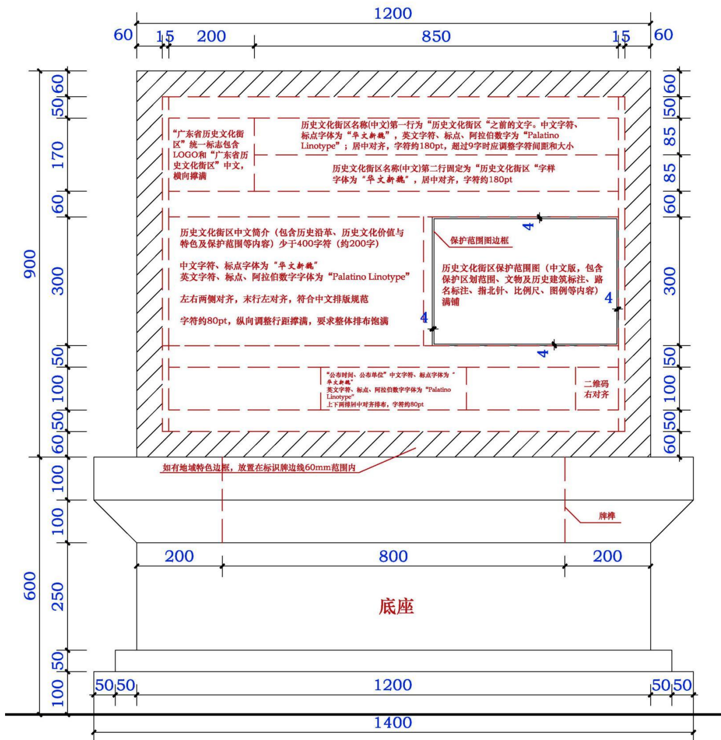
图 1: 保护标志牌排版规则、安装高度示意图 (横版正面)
