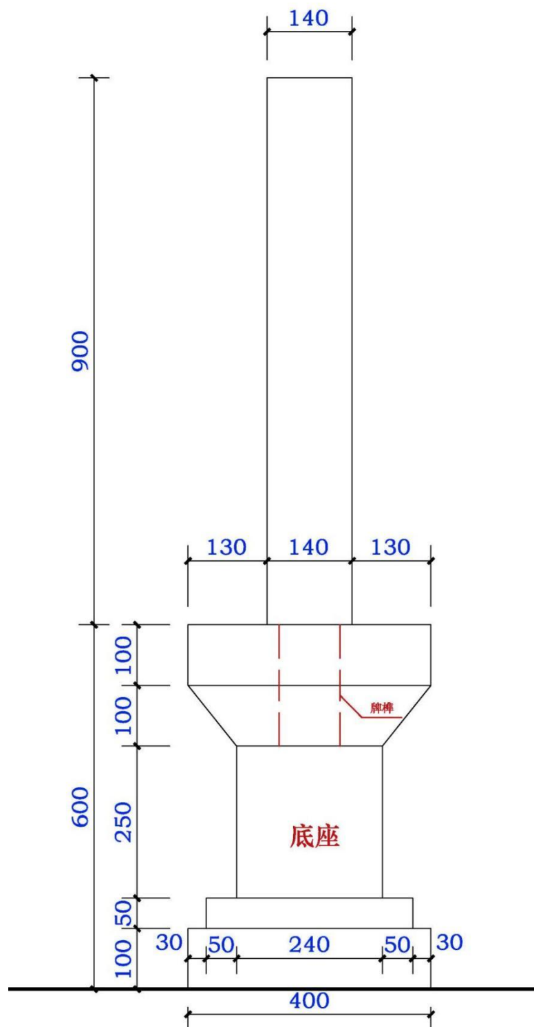
图 3: 保护标志牌排版规则、安装高度示意图（横版侧面）
