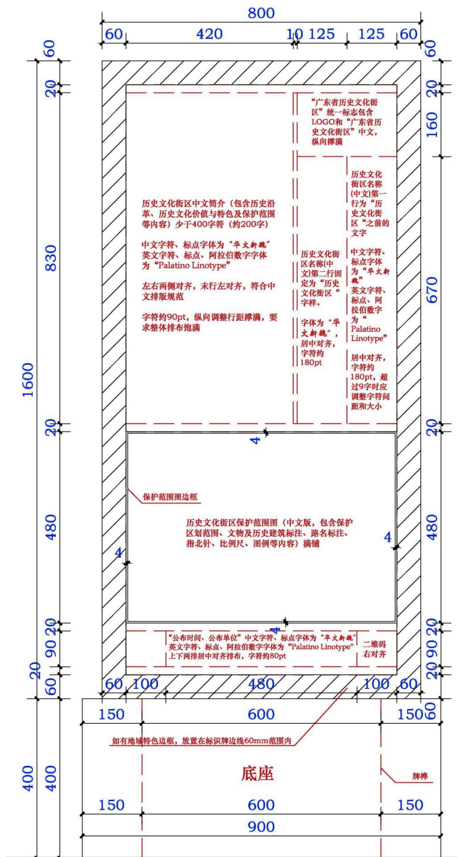
图 4: 保护标志牌排版规则、安装高度示意图 (竖版正面)
