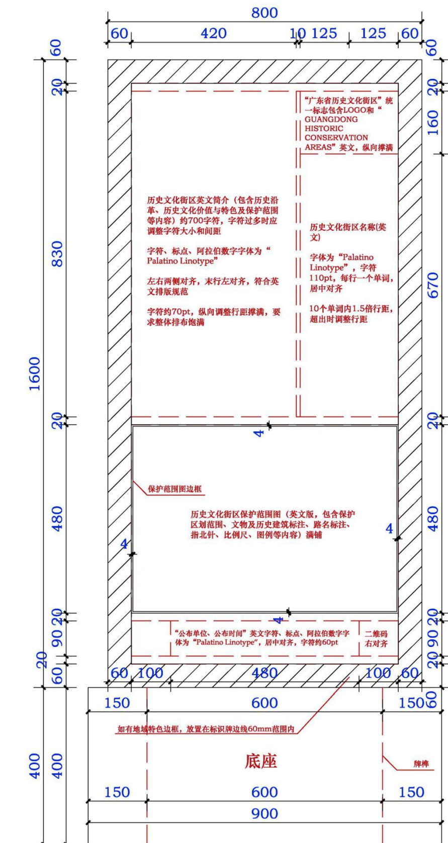
图 5: 保护标志牌排版规则、安装高度示意图 (竖版背面)
