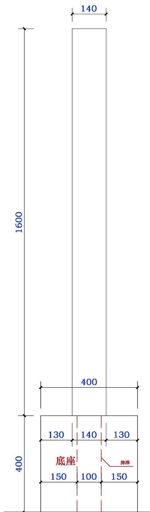
图 6：保护标志牌排版规则、安装高度示意图（竖版侧面）
